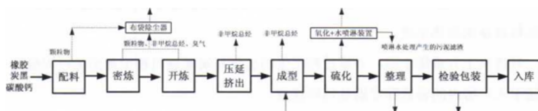
图 3-1 橡胶充气床垫生产工艺流程图
